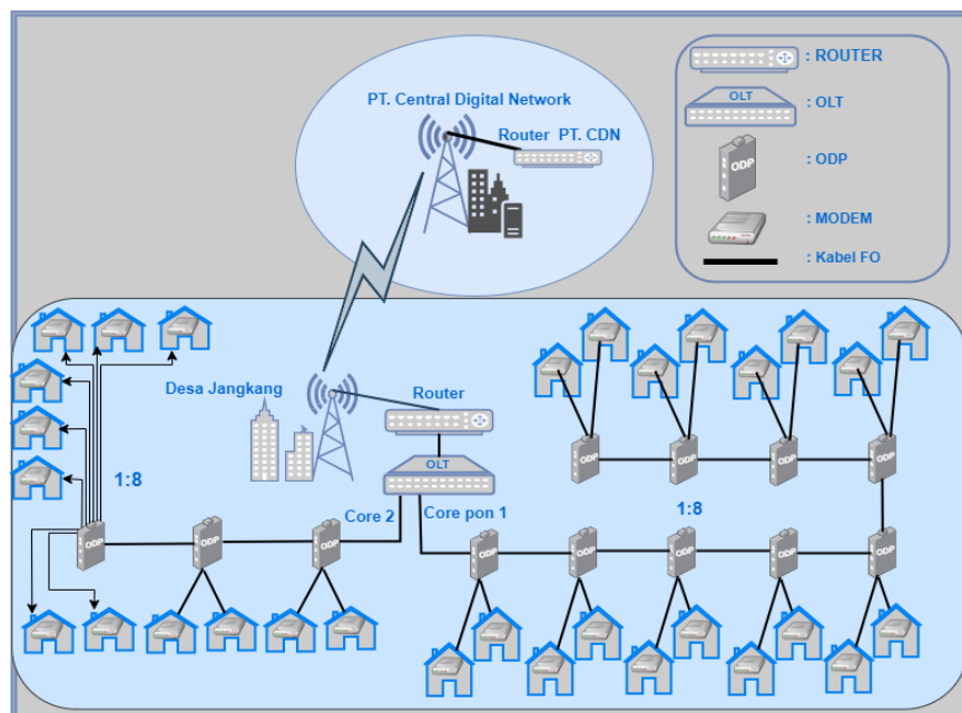
Gambar 4.10 Topologi jaringan FTTH Desa Jangkang
