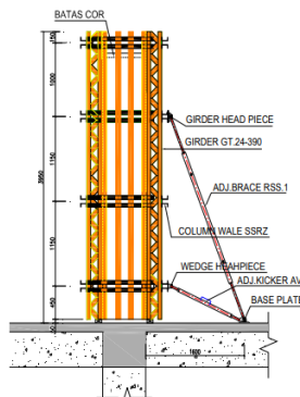
Gambar 3.24 Ilustrasi bekisting kolom lico peri Sumber : Dokumentasi lapangan
