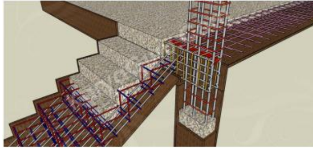
Gambar 3.28 Pekerjaan perakitan tulangan & pengecoran tangga
