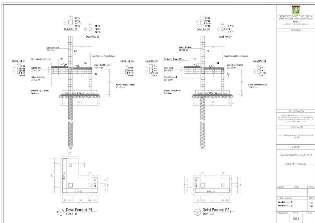
Gambar 3.27 Denah Pondasi P1 Dan P2 (Sumber: Dokumen Proyek)
