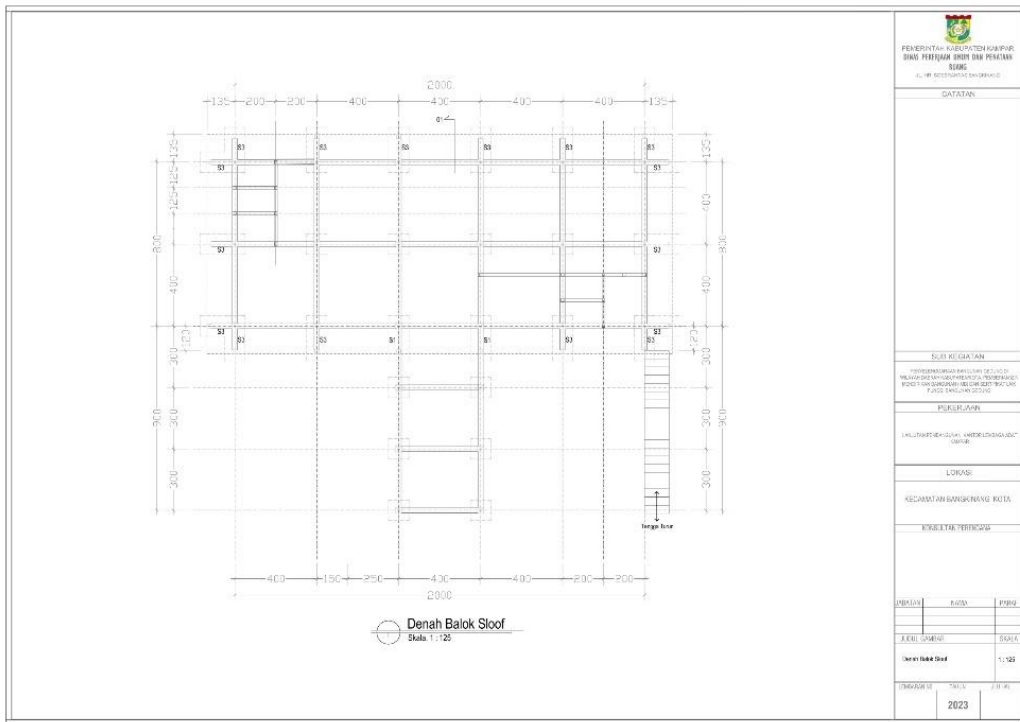
Gambar 3.26 Denah Balok Sloof (Sumber: Dokumen Proyek)
