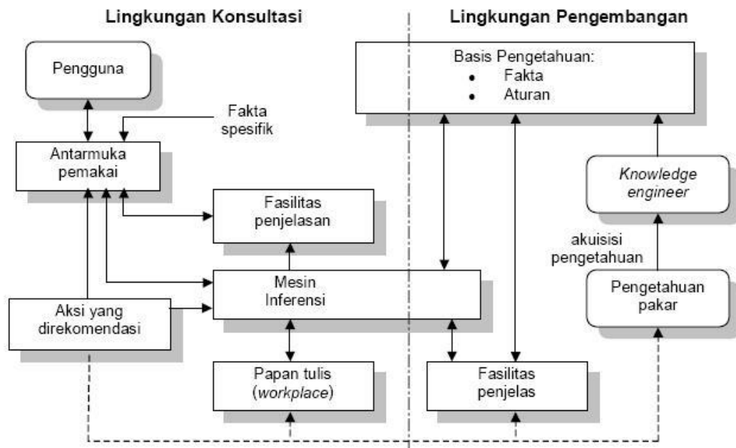
Gambar 2. 1 Arsitektur Sistem Pakar (Sumber: Buku Arsitektur Sistem Pakar)
