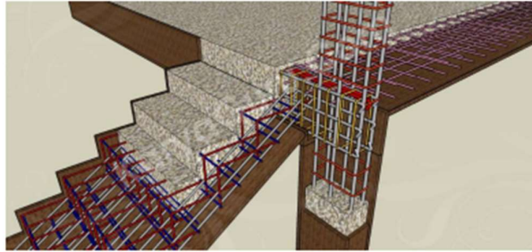
Gambar 3.28 Pekerjaan perakitan tulangan & pengecoran tangga Sumber : Ilustrasi metode pelaksanaan proyek
