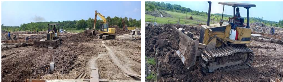
Gambar 3.5 Proses pemerataan jalan.
