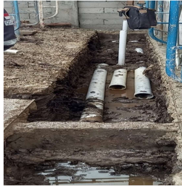
Gambar 3.41 Pekerjaan pemasangan pipa saluran air Sumber : Dokumentasi lapangan
