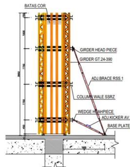
Gambar 3.24 Ilustrasi bekisting kolom lico peri Sumber : Dokumentasi lapangan
