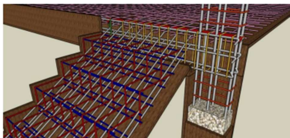
Gambar 3.27 Ilustrasi perakitan tulangan tangga Sumber : Ilustrasi metode pelaksanaan proyek
