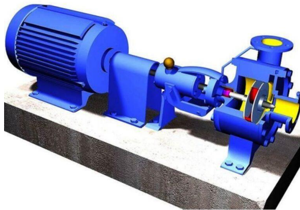
Gambar 1 3 pompa sentrifugal
