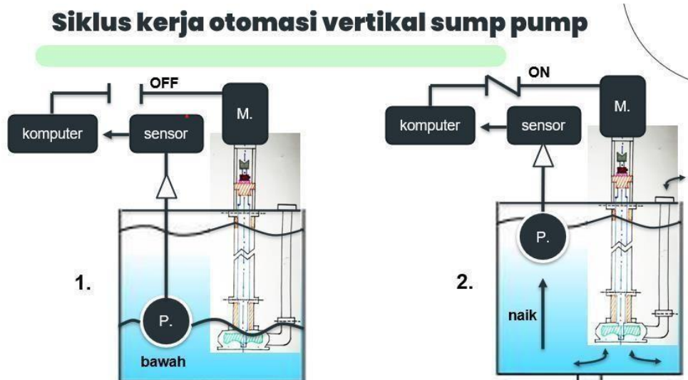
Gambar 4.4: gambar siklus otomasi vertikal sump pump
