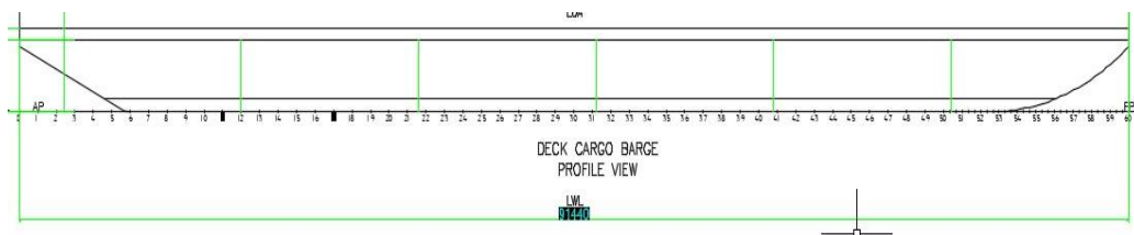
Gambar 2. 22 Mencari LWL
