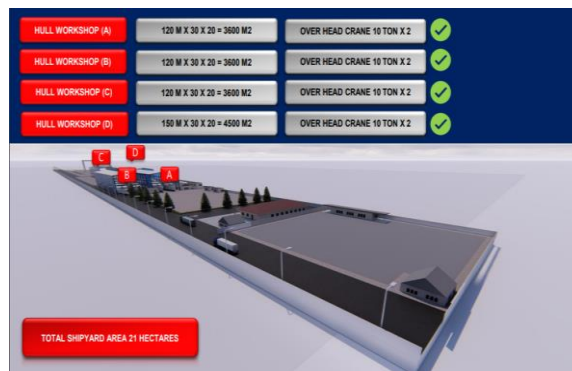
Gambar 1.3. Layout Galangan dan Bengkel-Bengkel
