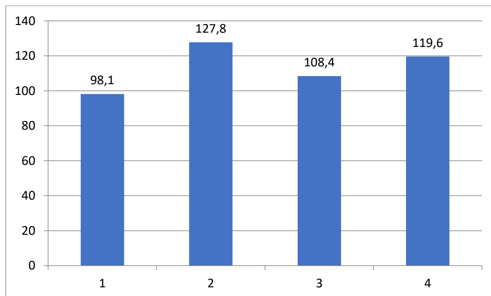
Gambar 4.3 grafik kuat Tarik kayu (Sumber: Pengolahan data Tugas Akhir, 2025)
