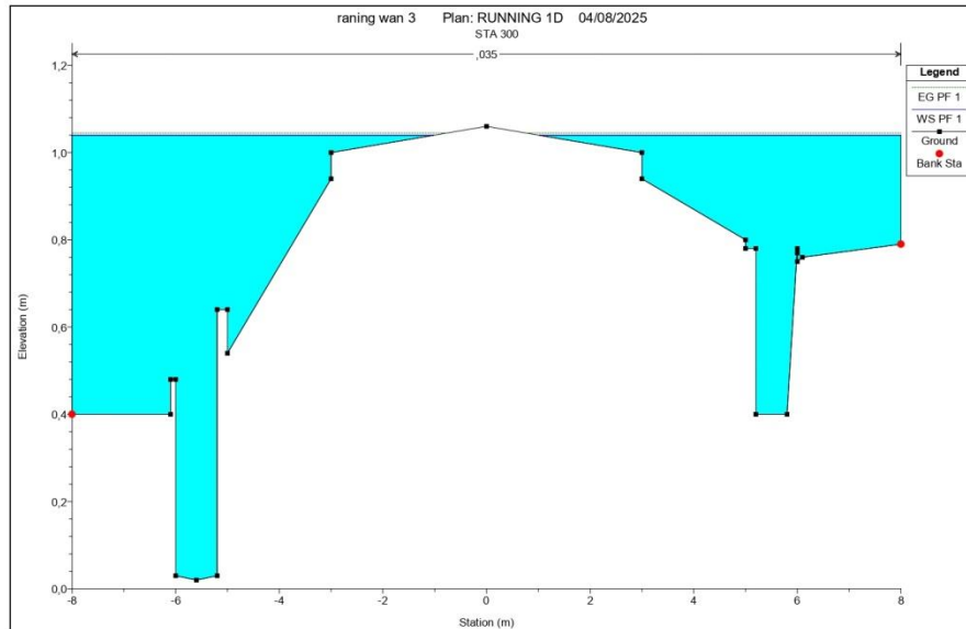
PENAMPANG SALURAN STA 0+300
