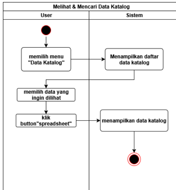
Gambar 4. 4 Activity Diagram Melihat & Mencari Data Katalog
