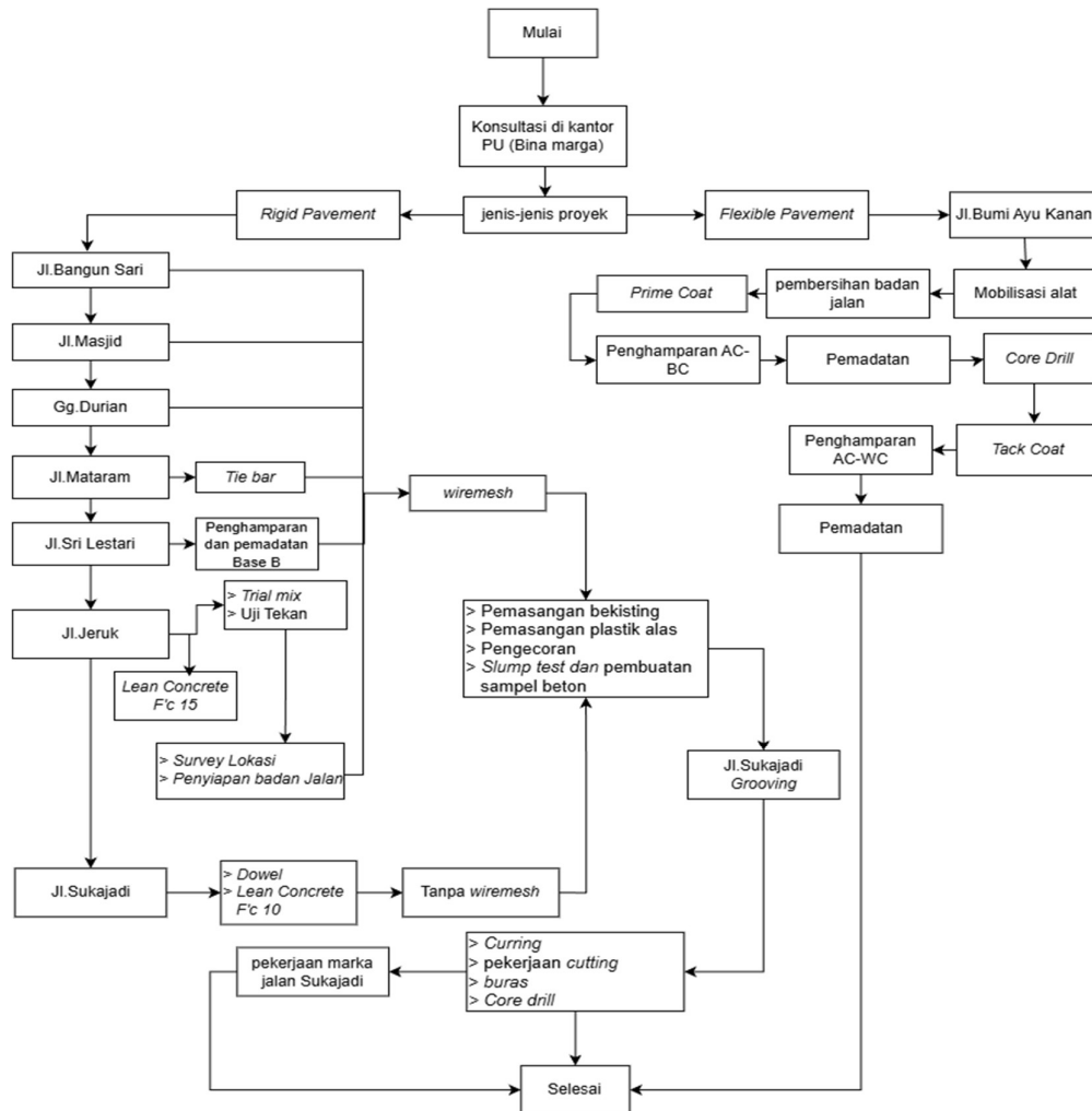
Gambar 1. 3 Flowchart lapangan
