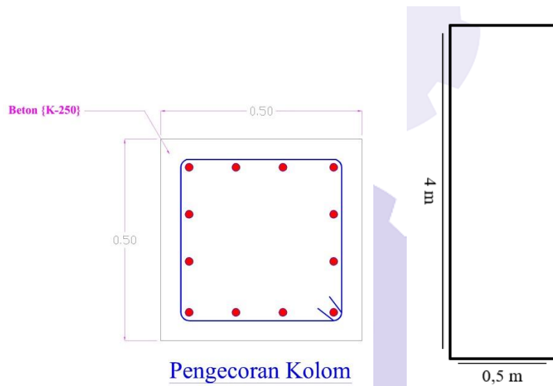
Gambar 3.33 Volume pengecoran
