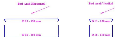
Detail Pembesian Peilcap
