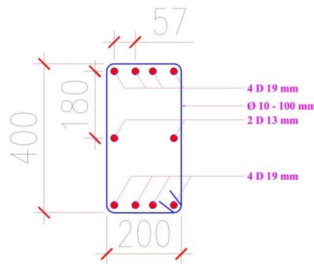
Gambar 3.49 Detail pembesian balok
