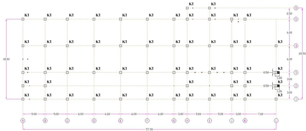
Denah Kolom
